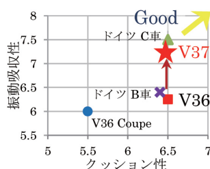
図-8 シート性能評価 Fig. 8 Seat evaluation
