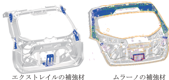
図-16 バックドアの補強構造 Fig. 16 Reinforcement of tailgate
