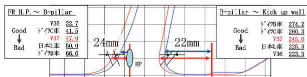
図-14 Bピラー位置の見直し Fig. 14 Change of B-pillar position
