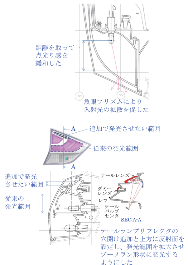
図-20 リヤシグネチャ光学構造 Fig. 20 Rear signature optical structure
