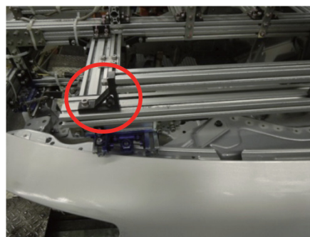
図-74 フロントフェンダ位置決め構造 Fig. 74 Front fender positioning jig structure
