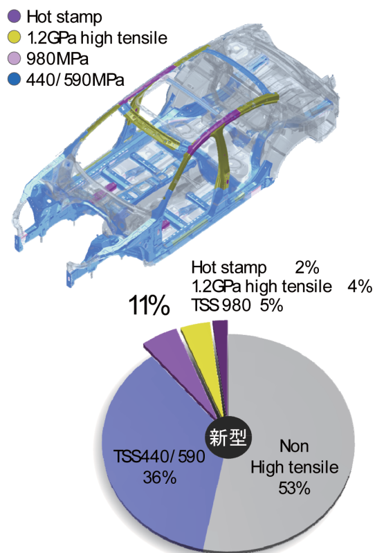
図-45 新型スカイライン（V37型）のハイテン材使用マップ Fig. 45 High tensile steel map
