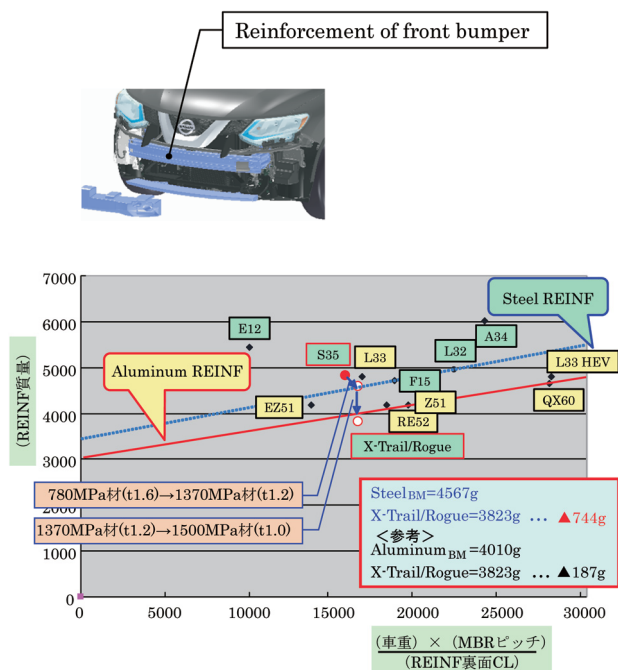
図-17 質量比較 Fig. 17 Mass comparison
