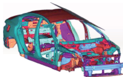
図-46 ルーフ圧壊（解析モデル） Fig. 46 Roof intrusion (CAE model)
