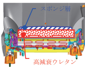
図-9 シート構造 Fig. 9 Seat structure
