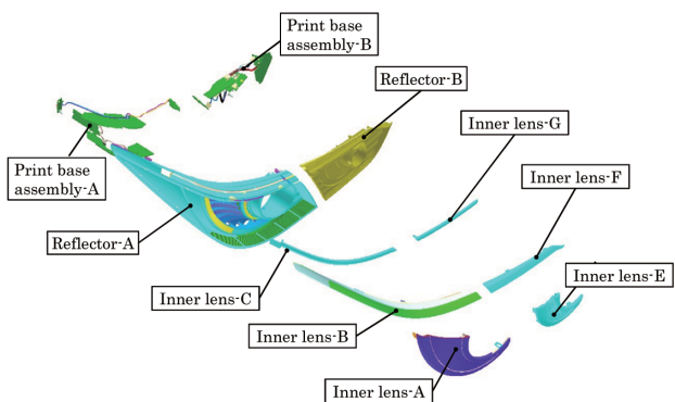
図-42 リヤコンビネーションランプ内部構造
