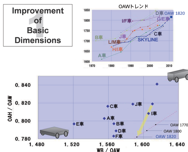
図-12 基本諸元の競争力指標の例 Fig. 12 Index example of major dimension comparison
