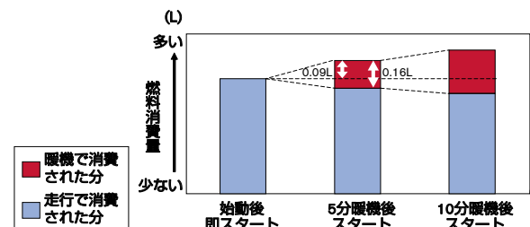
暖機による燃料消費量の変化 気温25℃で市街地走行4.2km
